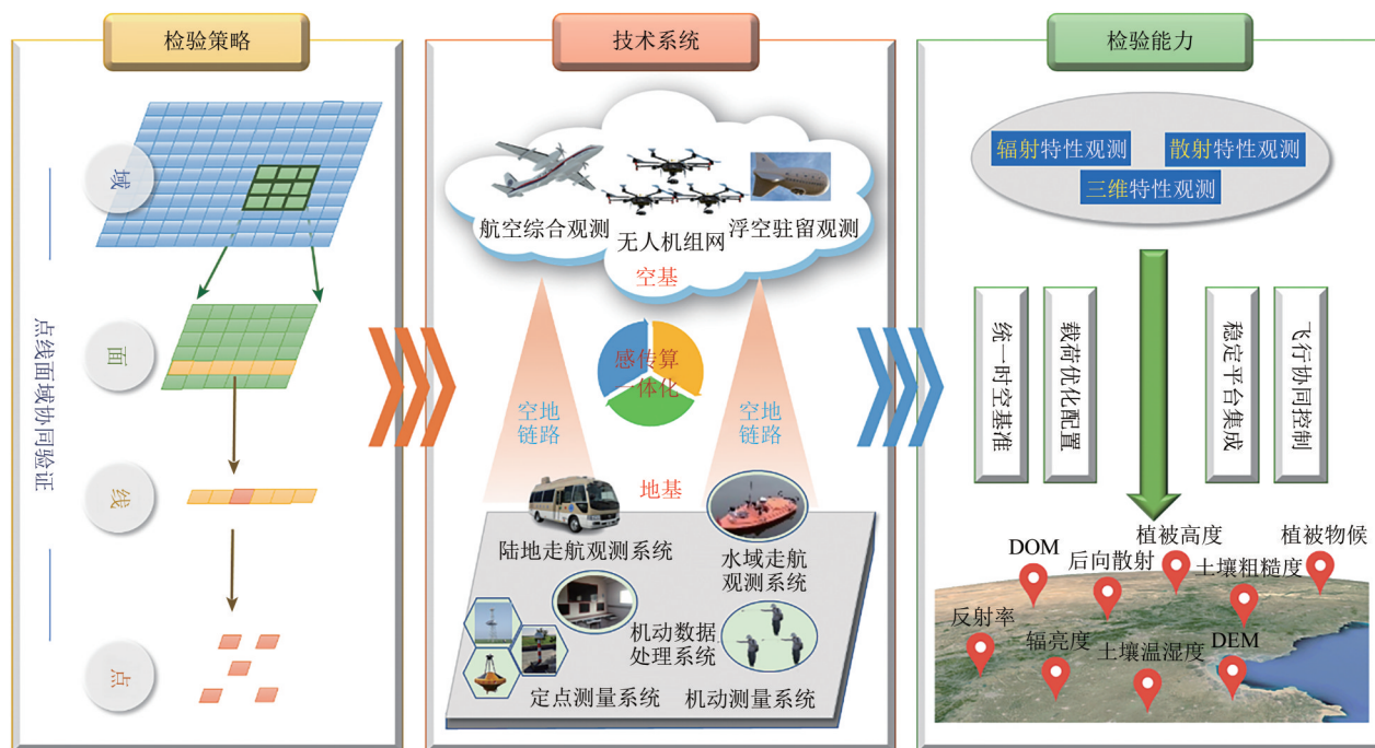
图5 航空协同真实性检验系统组成
